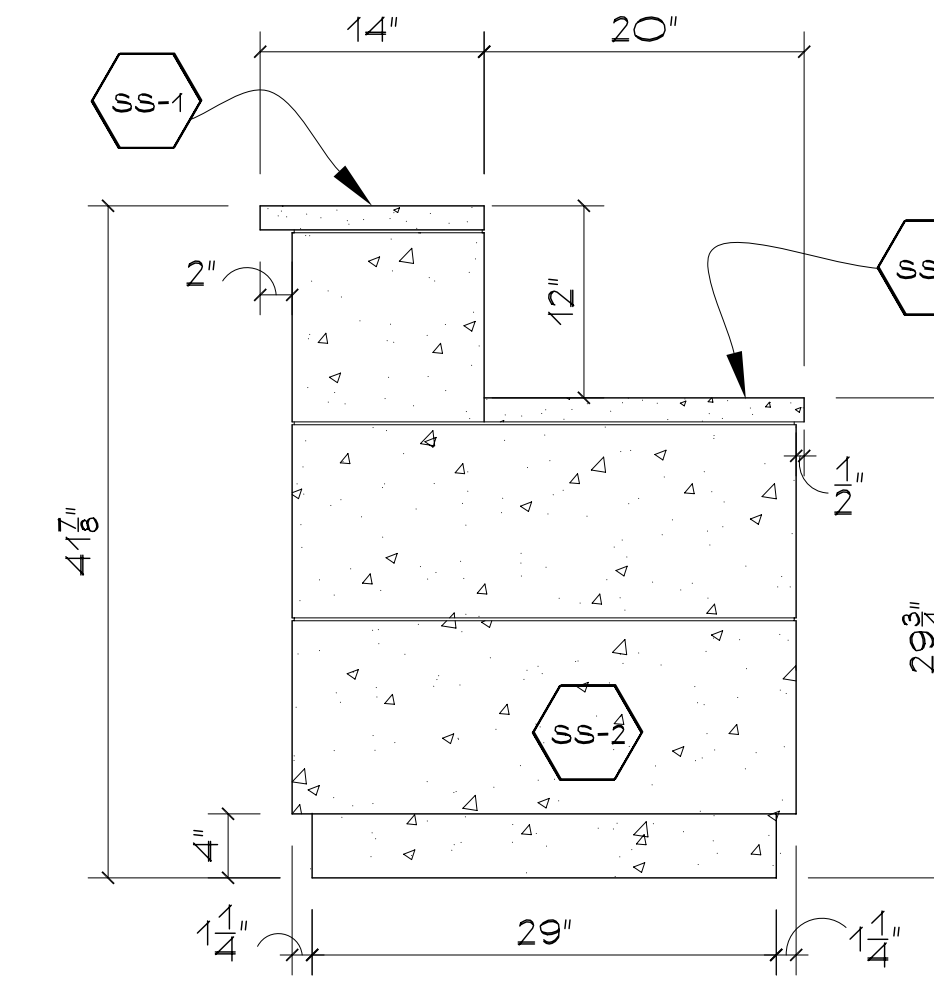
3 ELEVATION SC. 1/4"=1'-0"
