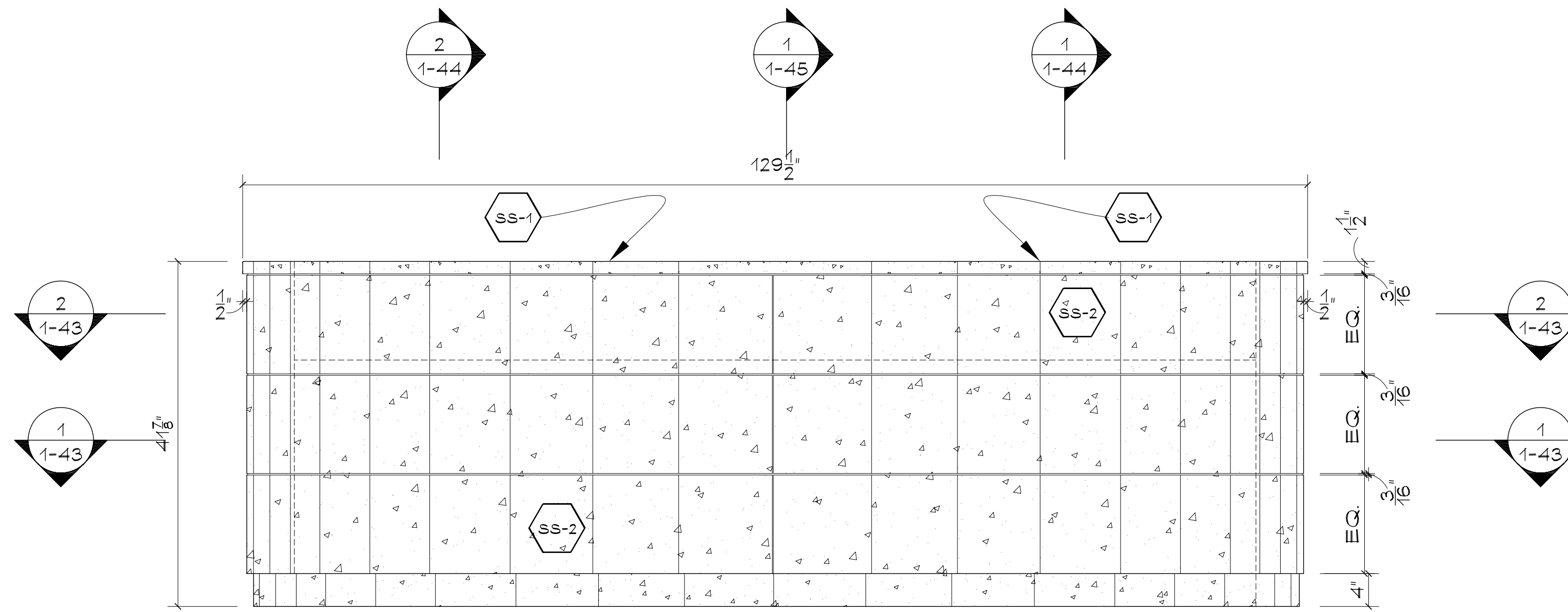
2 ELEVATION SC. 1/4"=1'-0"
