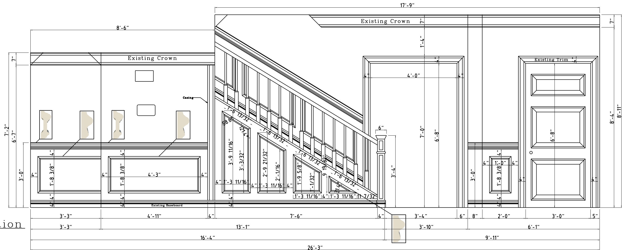
B Elevation
