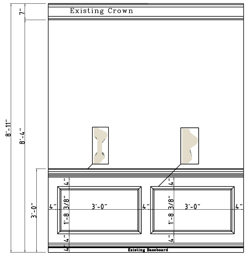
E Elevation
