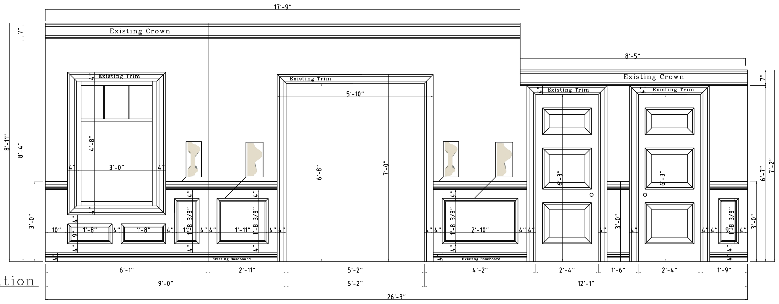
E Elevation
